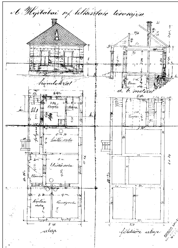
A lelkészlak tervrajza 1914-ből
