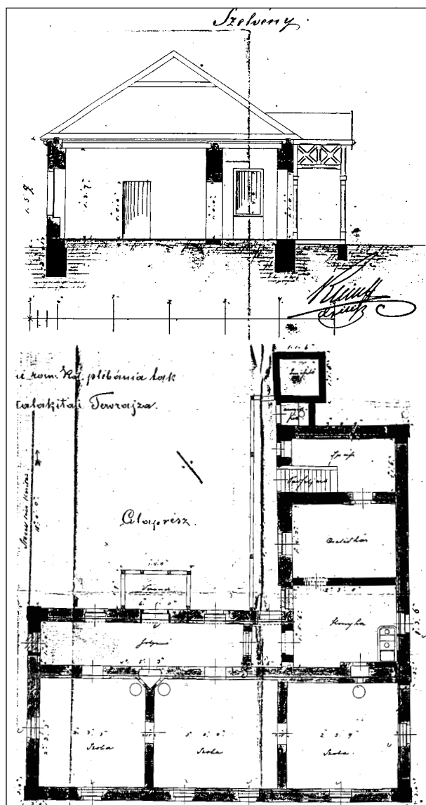
A katolikus parókia tervrajza és nézete 1880-ból (E. É. Lt. AN. r. sz. 1083. 130/1880.)
